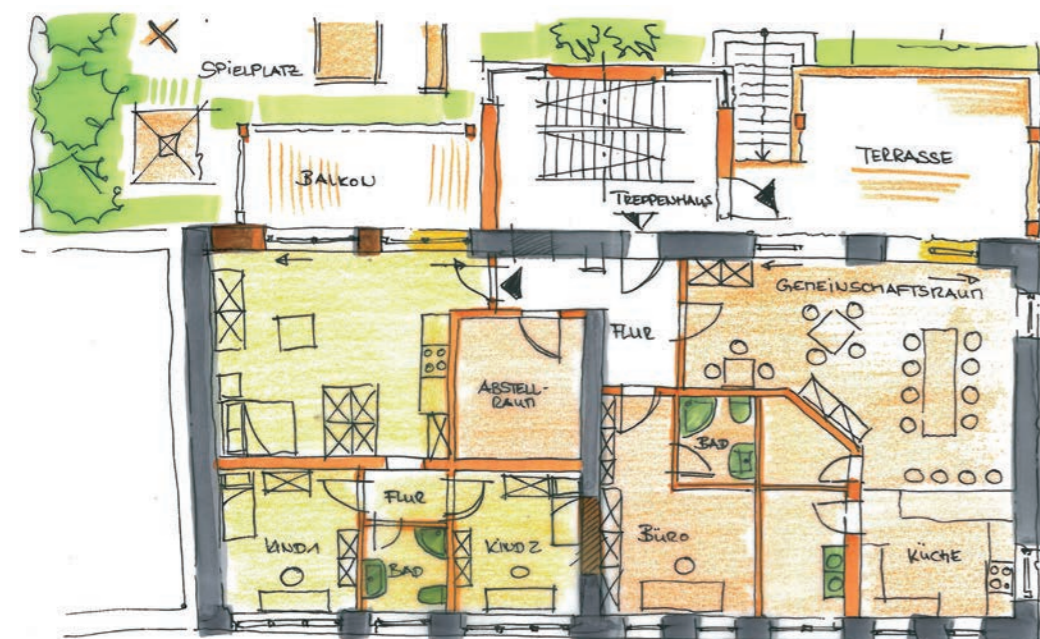
Erdgeschoss Apartment mit Gemeinschaftsräumen
